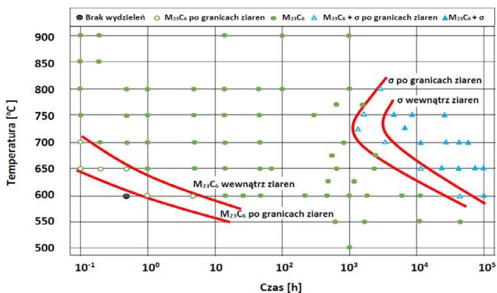
Rys. 1. Wykres CTW zakresów wydzielenia faz wtórnych w stali Super 304H [19]
