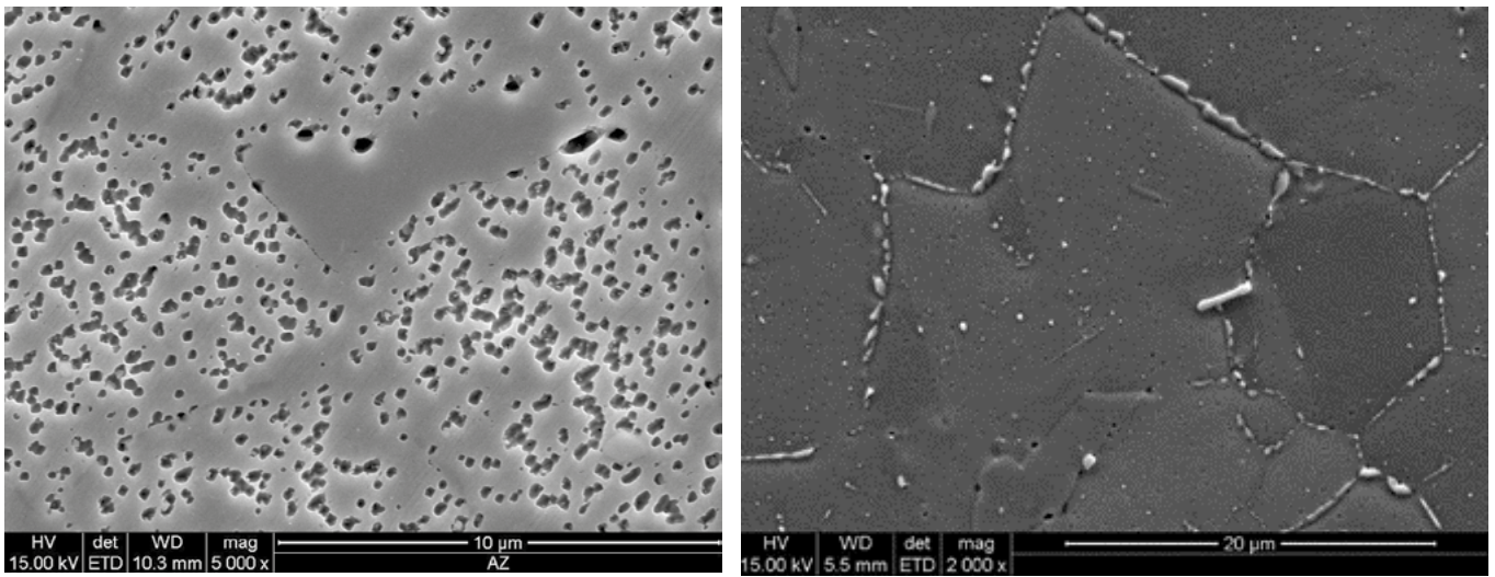
Rys. 6. Mikrostruktura stali Super 304H po starzeniu w temperaturze 700°C/20 000 godzin z wydzieleniami fazy \epsilon -Cu w osnowie oraz węglików M23C6 i fazy \sigma po granicach ziaren, obserwacja SEM
