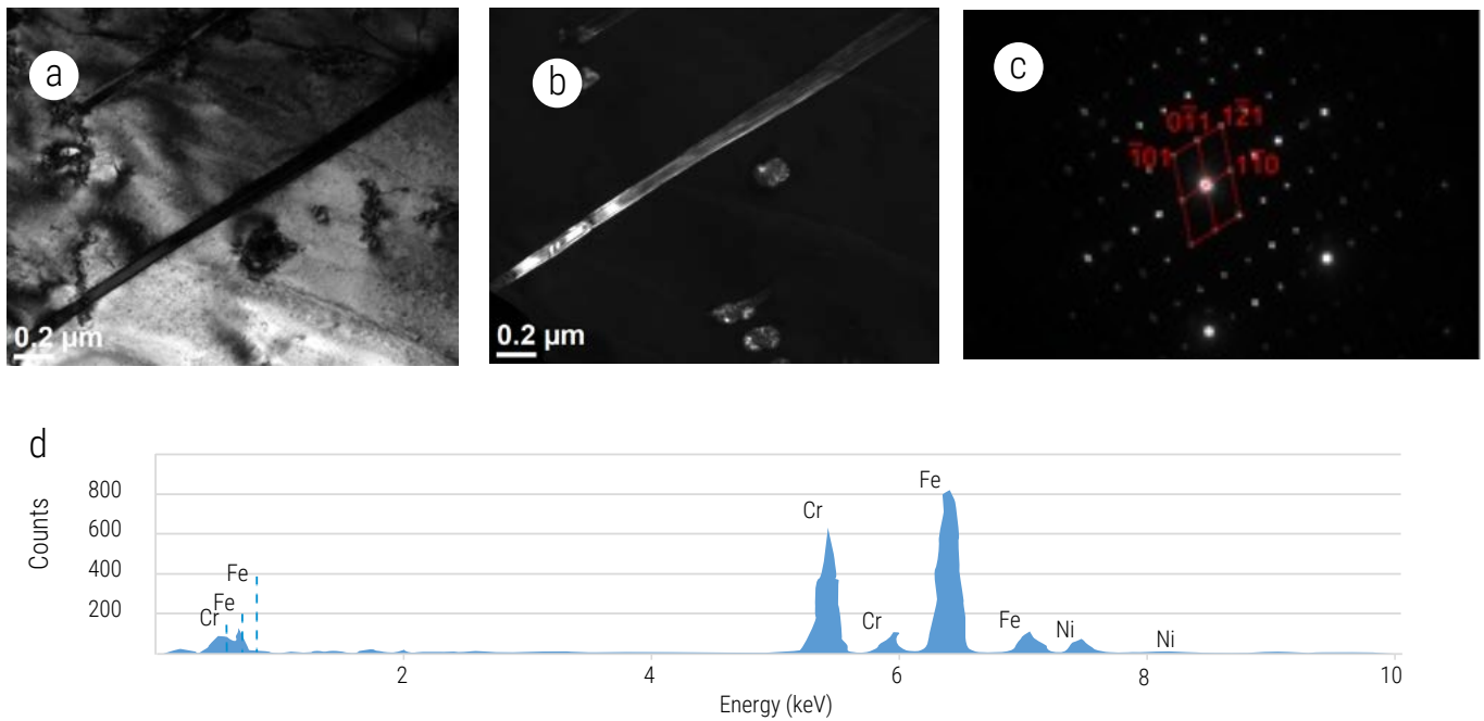
Rys. 9. Wydzielenia w stali S304H po starzeniu w temperaturze 700°C przez 20 000 godzin: a) fazy \sigma , b) fazy \sigma , c) dyfraktogram fazy \sigma , d) analiza EDS. Obserwacja TEM
