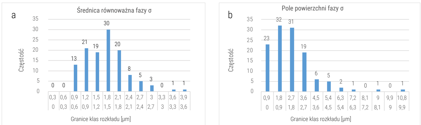
Rys. 4. a) Wyniki analizy ilościowej średnicy równoważnej wydzieleni fazy \sigma po 20 000 godzin starzenia w temperaturze 650°C (min – 0,65 max – 3,7), b) Wyniki analizy ilościowej wydzieleni pola fazy \sigma po 20 000 godzin starzenia w temperaturze 650°C (min. – 0,33 max. – 10,74)
