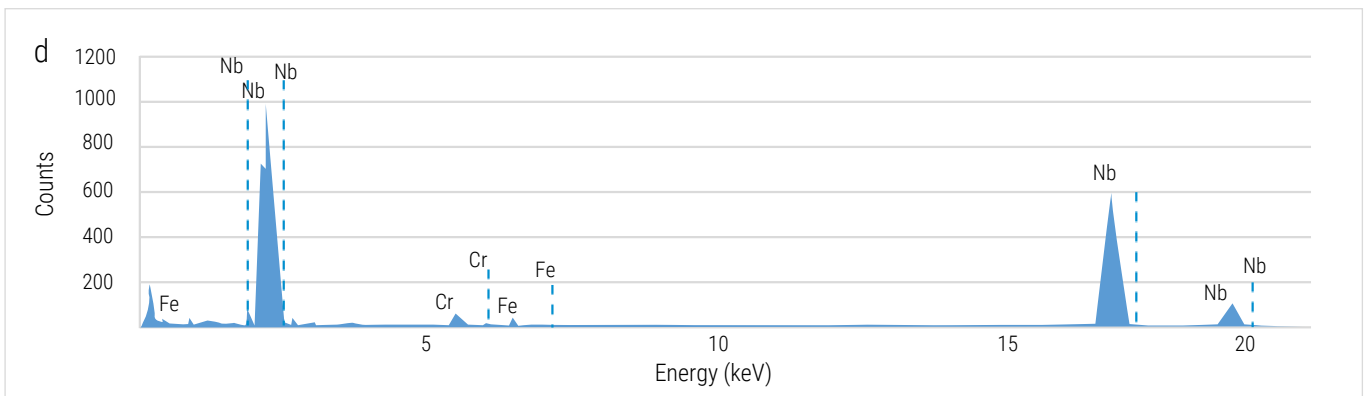
Rys. 5. Wydzielenia w stali S304H po starzeniu w temperaturze 650°C przez 20 000 godzin a), b) wydzielenie MX, c) dyfraktogram MX, d) analiza EDS. Obserwacja TEM
