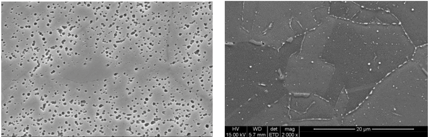
Rys. 3. Mikrostruktura stali Super 304H po starzeniu w temperaturze 650°C/20 000 godzin z wydzieleniami fazy \epsilon -Cu w osnowie oraz węglików M_{23}C_6 i fazy \sigma po granicach ziaren, obserwacja SEM
