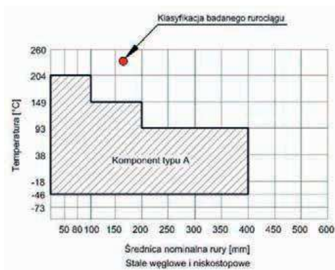
Rysunek 3. Kategoriezacja komponentów typu A
