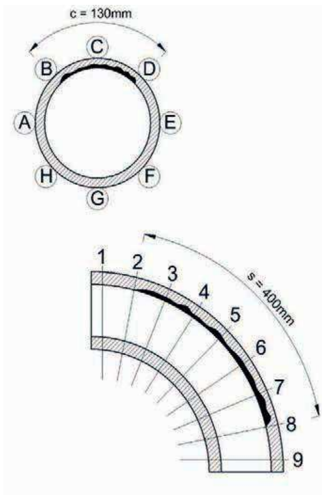
Rysunek 2. Schematyczne przedstawienie zasięgu występowania lokalnego ubytku korozyjnego
