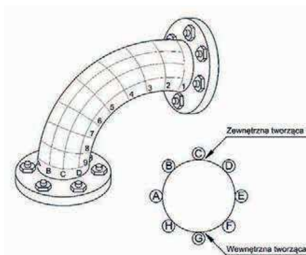
Rysunek 1. Schemat siatki pomiarowej wykorzystanej podczas badań
